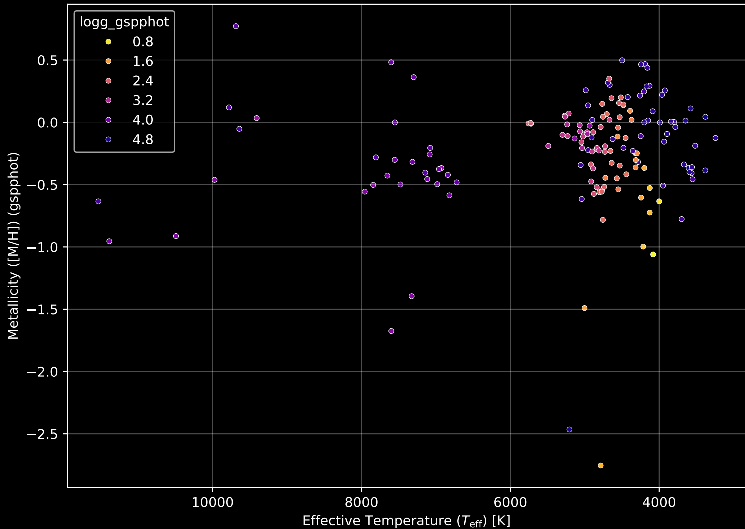
APOGEE DR17 Field: [TRIAND-5] Stellar Population Parameters (n= 153)
